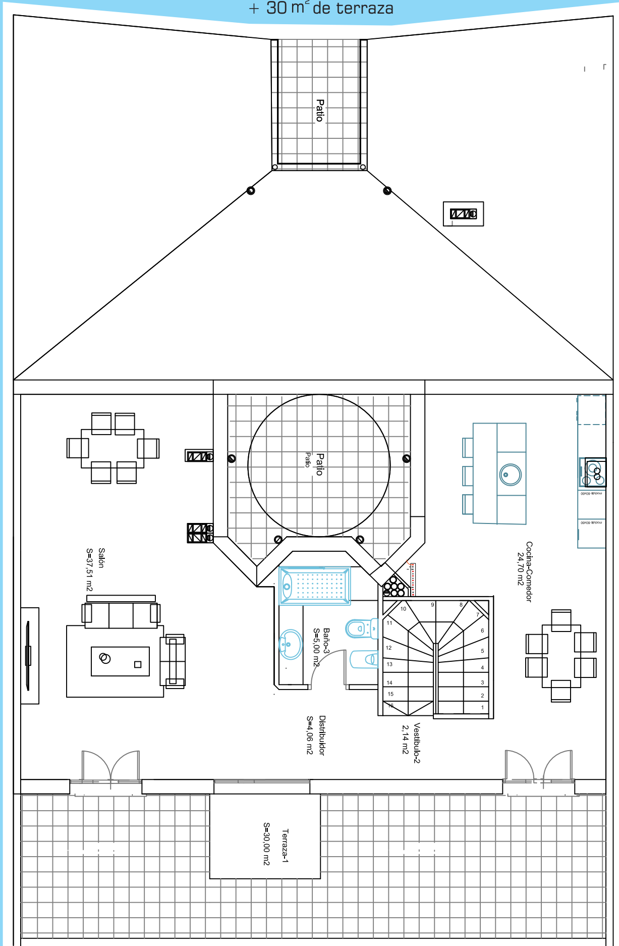
PLANTA TIPO 4º A - DUPLEX
